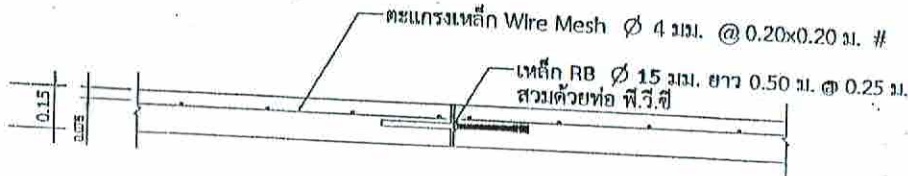
EXPANSION JOINT(ทุกๆระยะ 100.00 เมตร)
