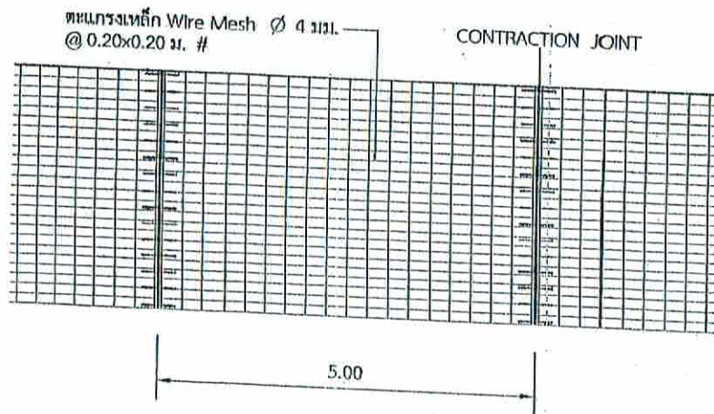
แปลนแสดงการเสริมเหล็กถนน ค.ส.ถ.
