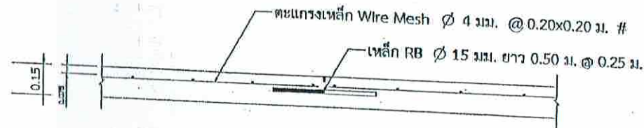
CONTRACTION JOINT(ทุกๆระยะ 5.00 เมตร)
